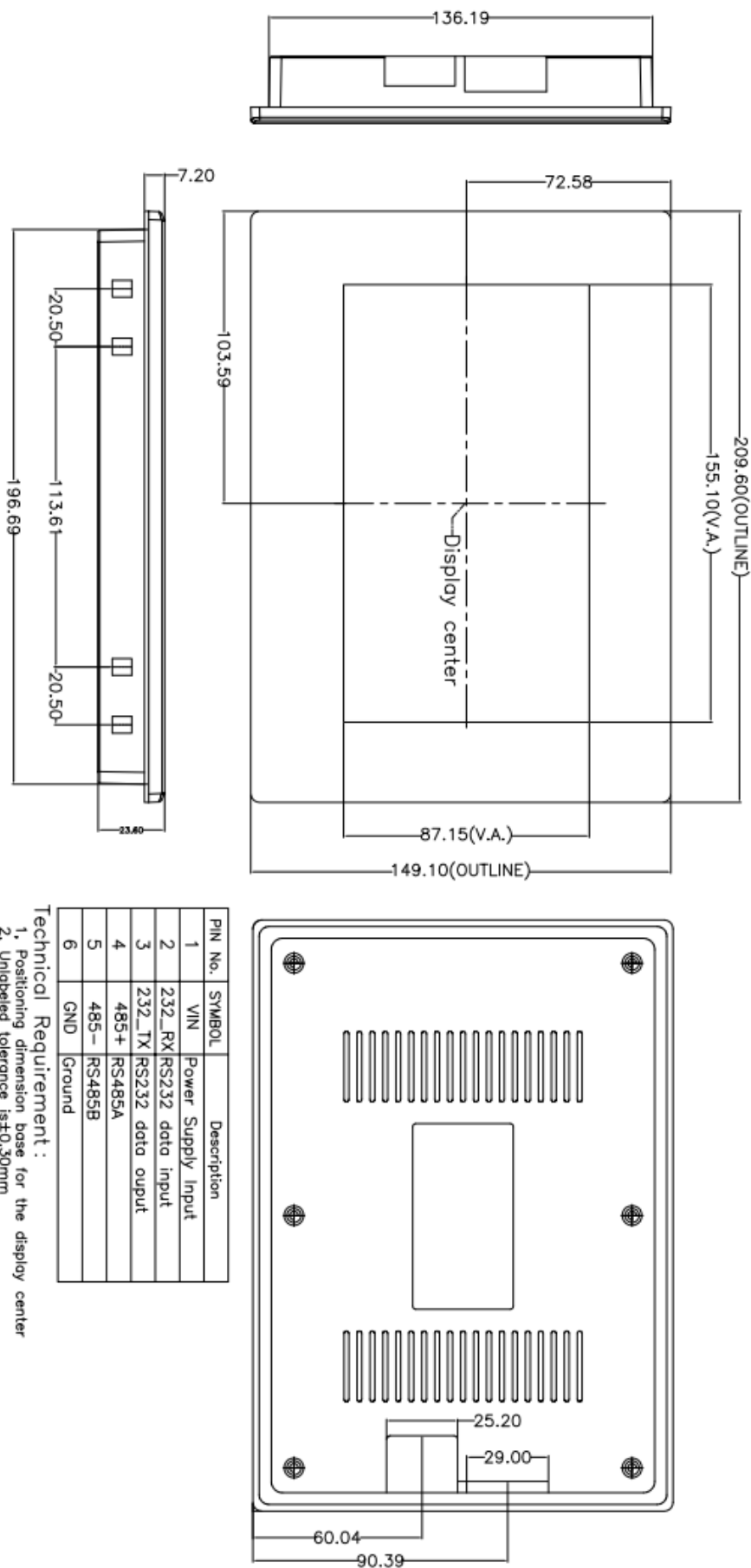
产品尺寸图(单位 mm , 未注公差±0.3mm)
